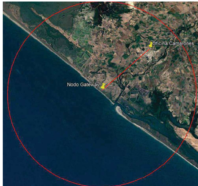
Figura 14. El círculo en rojo representa el hipotético alcance de lora de 15Km, la línea roja representa la distancia de 10Km que existe entre las oficinas de camarones y los estanques acuícolas en donde se encuentra el Gateway.
