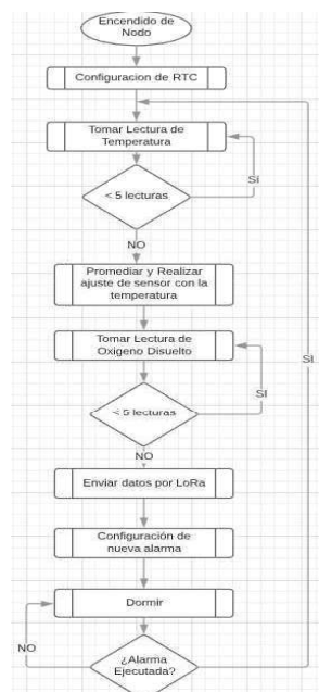
Figura 6. Diagrama de flujo del nodo de monitoreo
