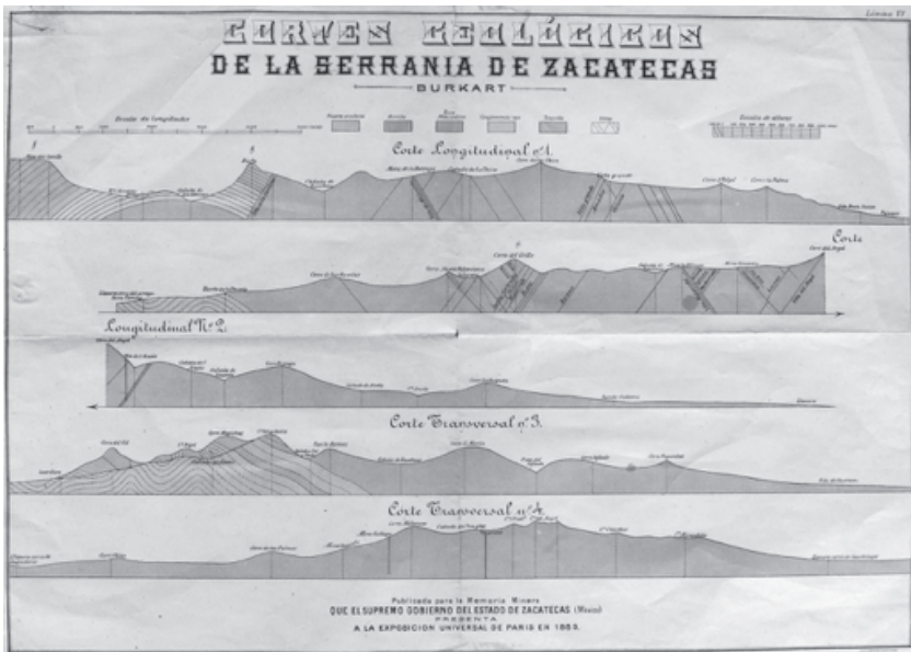
2815.- Plano Cortes Geológicos de la Serranía de Zacatecas, Burkart, Exposición Universal de París, 1889, Colección de Bernardo del Hoyo.
